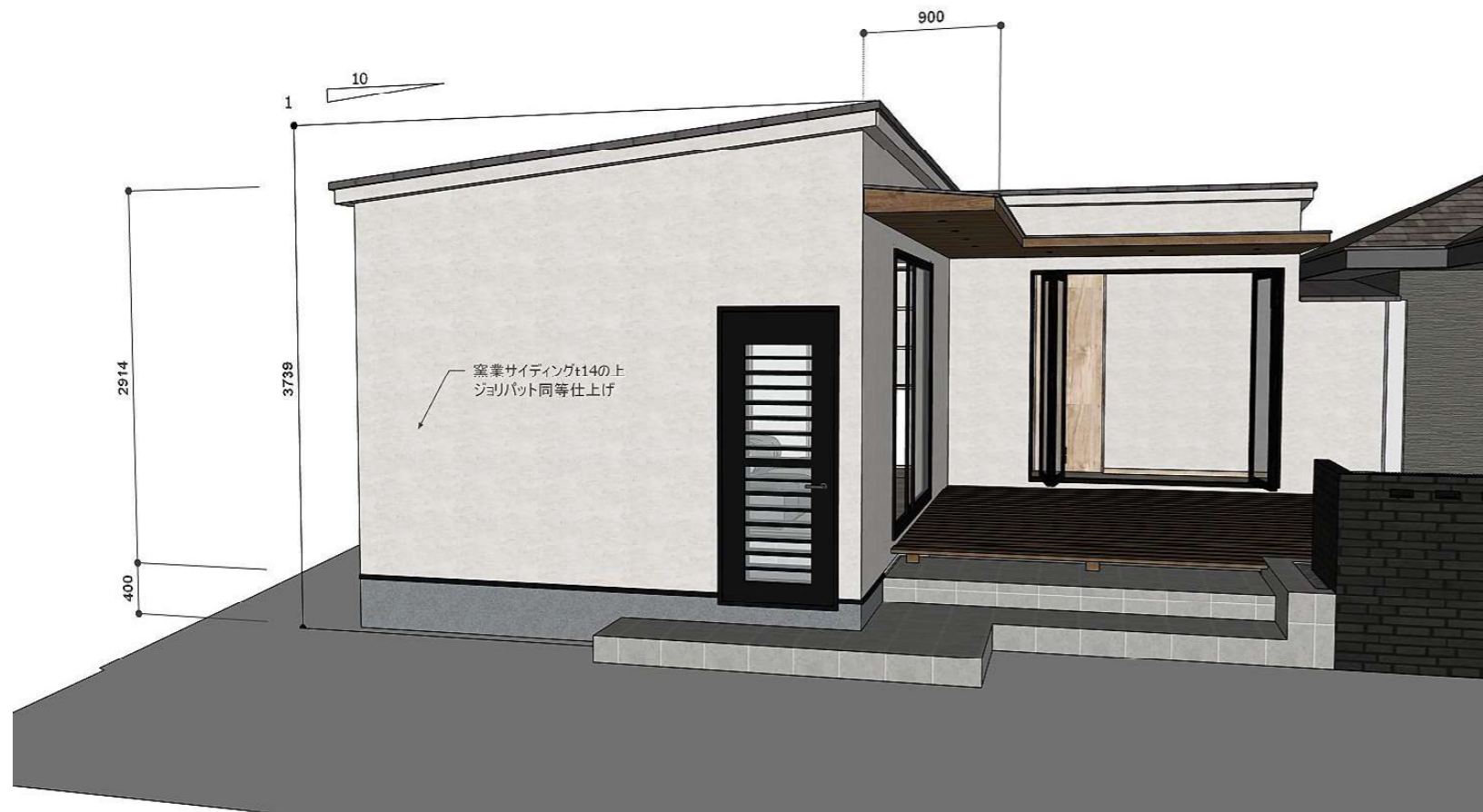
建物高さ(正面)
